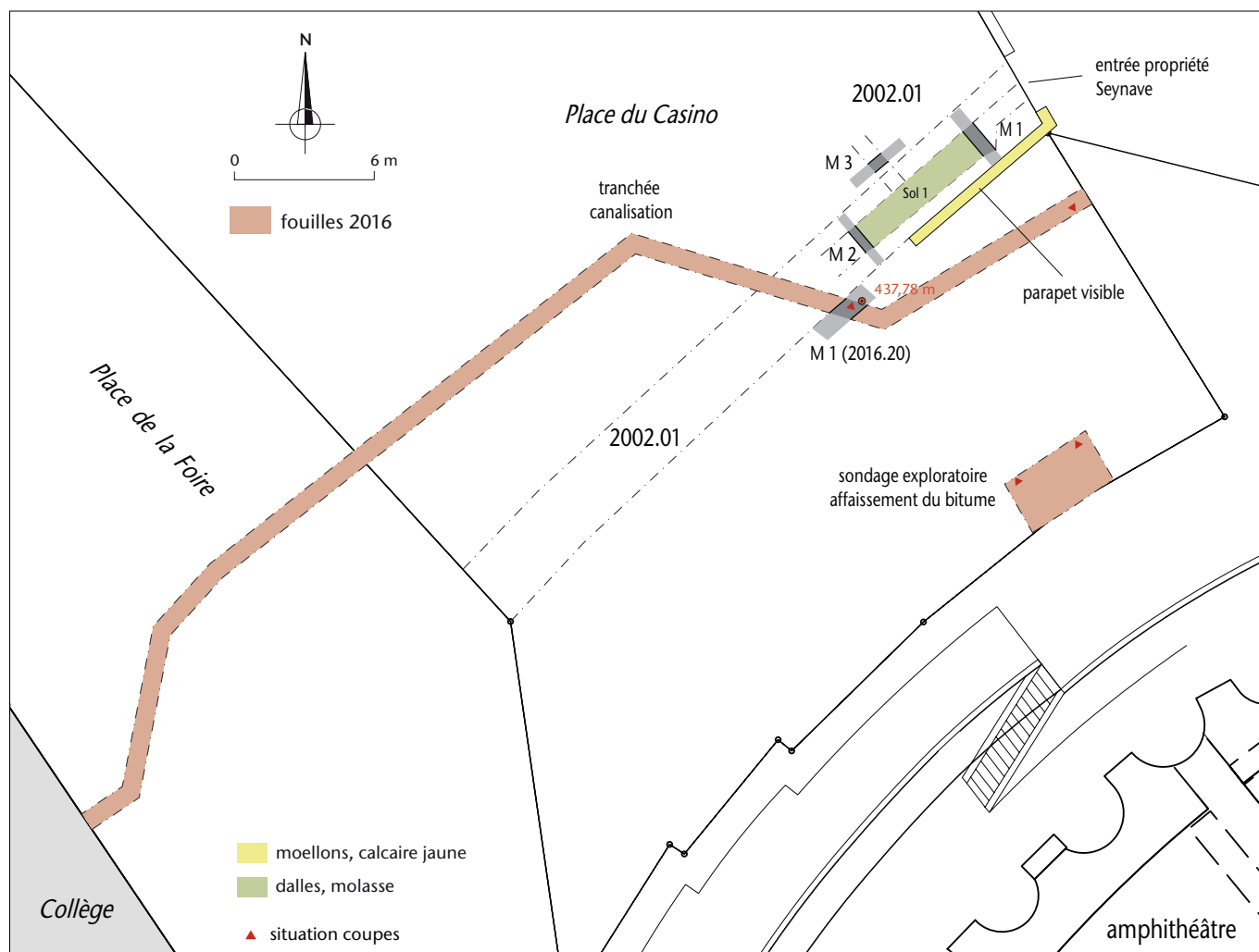
Fig. 95 2016.20. Place du Casino. Plan des vestiges fouillés en 2016 et en 2002.
