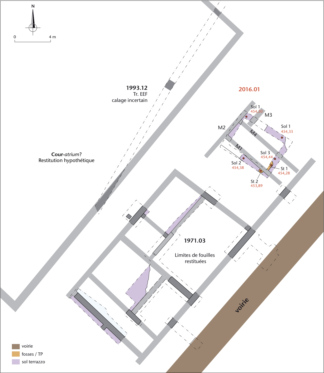
Fig. 9 2016.01. Chemin Derrière-la-Tour 2. Plan des vestiges fouillés en 2016 et restitution hypothétique des maçonneries mises au jour lors d'anciennes interventions (1971 et 1993).
