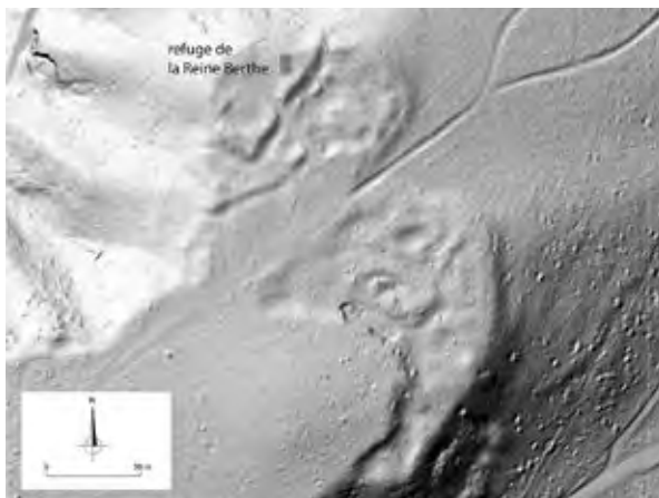
Extrait du modèle numérique de terrain (MNT) du Bois de Châtel. Ce type de documents reproduit avec une grande précision la microtopographie du sol. Les zones d'extraction du grès sont parfaitement perceptibles sous la forme de creux et d'amas irréguliers. Une petite fortification rectangulaire de datation incertaine est aussi visible au niveau du refuge de la Reine Berthe (en haut de l'image).
