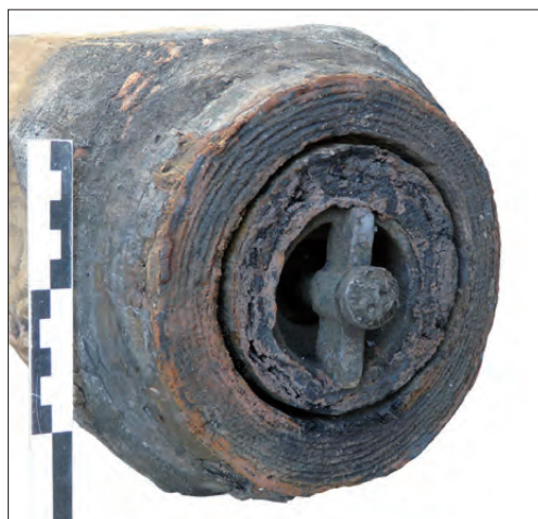
Fig. 28 (à g.) 2010.03. Place de l'Église. Détail de la soupape présente à la base de la conduite.
