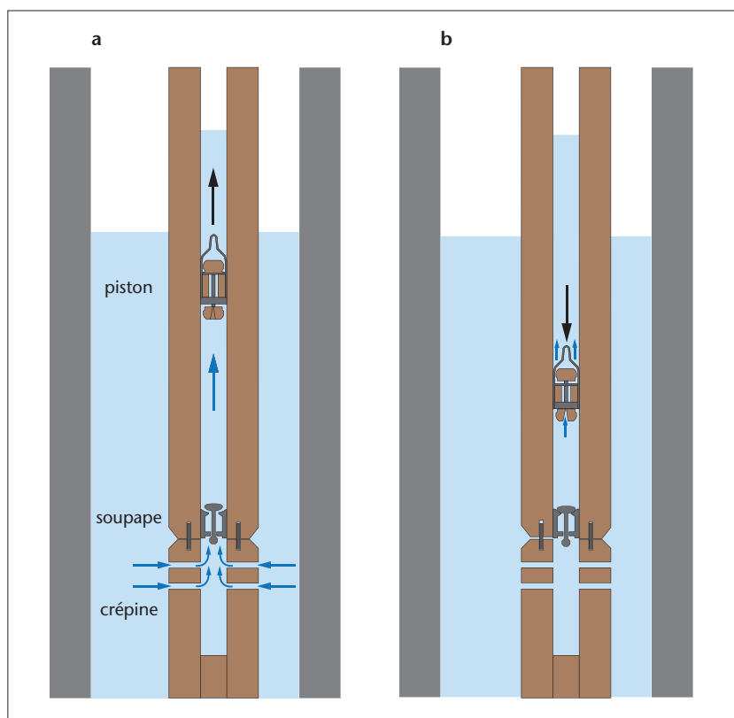
Fig. 30 2010.03. Place de l'Église. Fonctionnement du système de pompage que l'on peut restituer pour le puits.
